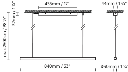
BLOKINLINE LEDTUBE S 900
